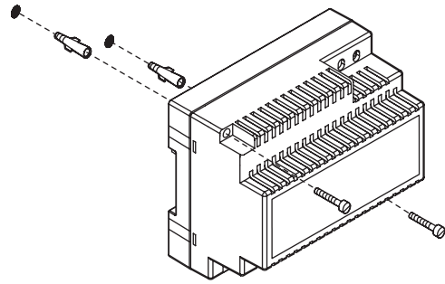
Instalación con apoyo de pared
