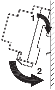
Instalación en barra DIN (6 módulos de 18 mm)
