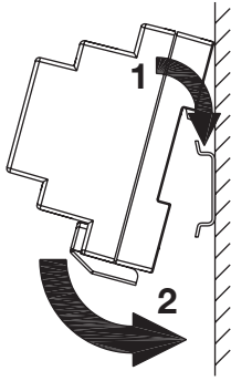
Installation on DIN bar (6 modules, 18 mm)
