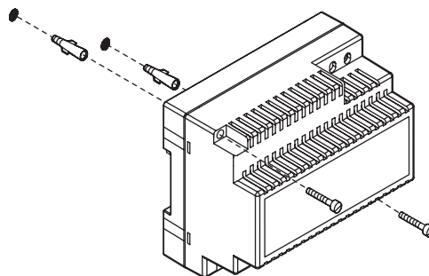
Installazione ad appoggio parete
