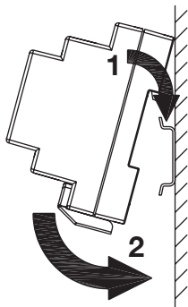
Installation sur barre DIN (6 modules de 18 mm)
