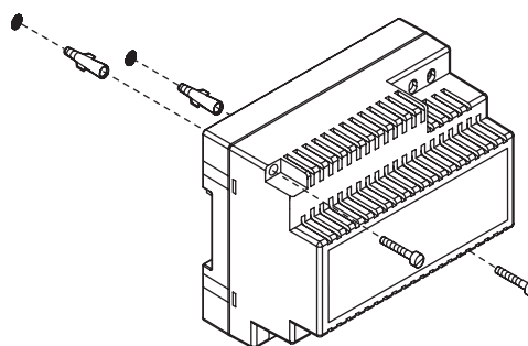
Installatie tegen de wand
