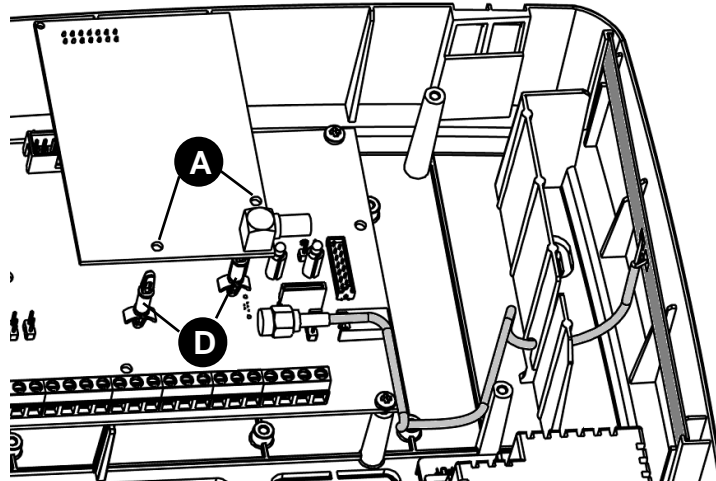
Zentrale 1068/005
