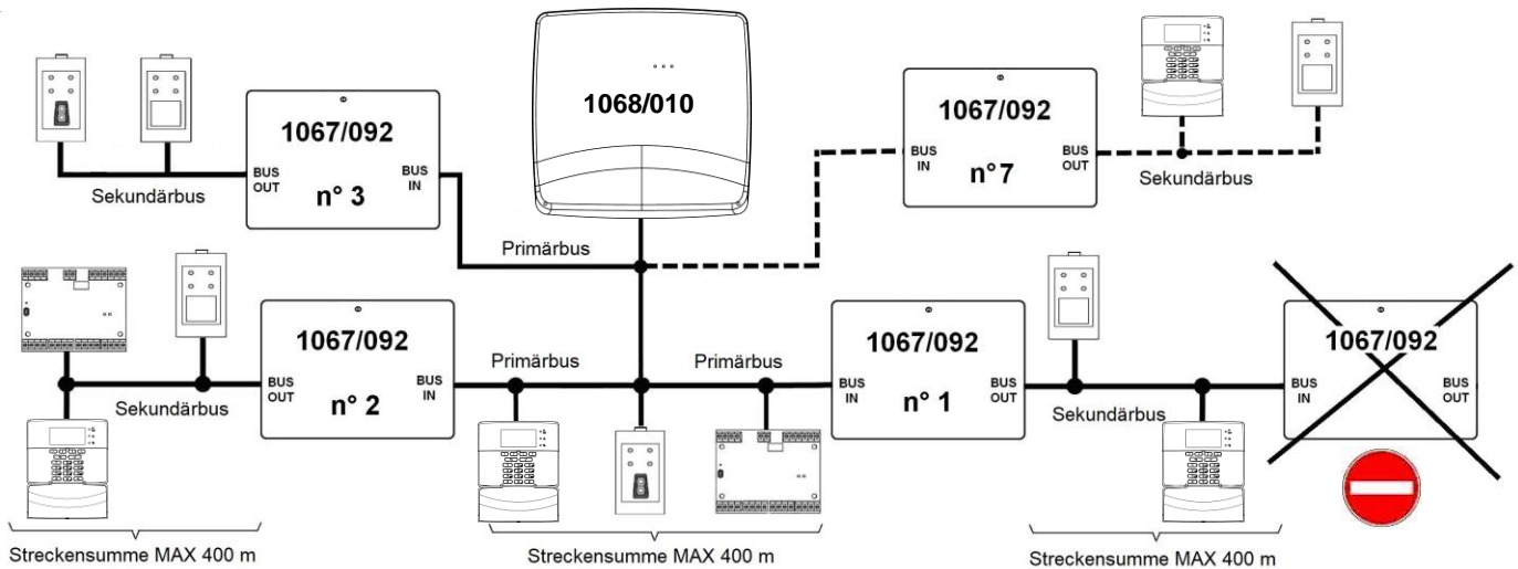
Abbildung 7 - Schema mit 7 zusätzlichen Netzteil-Repeatern
