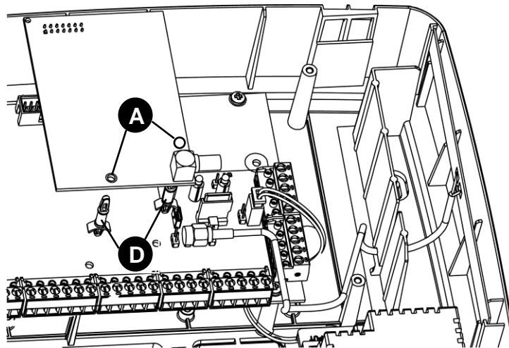
Zentrale 1068/010
