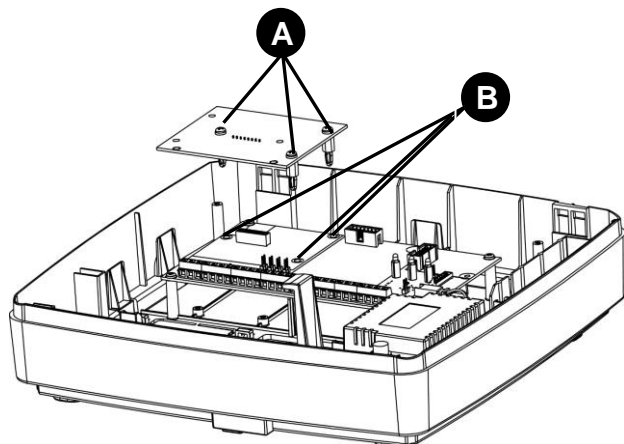
Zentrale 1068/005
