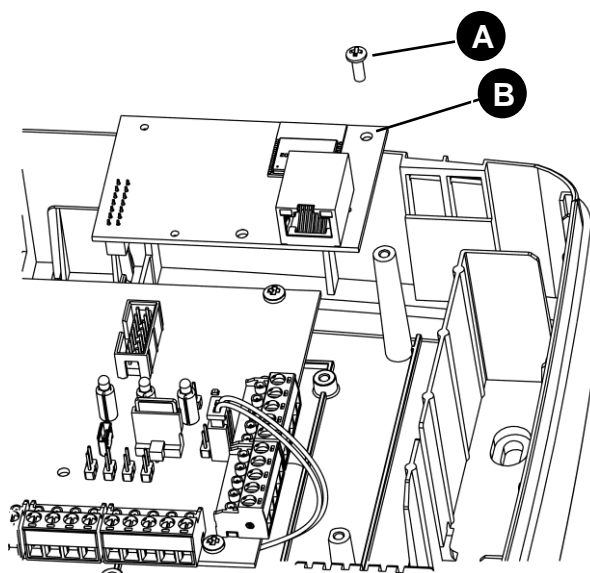
Zentrale 1068/010
