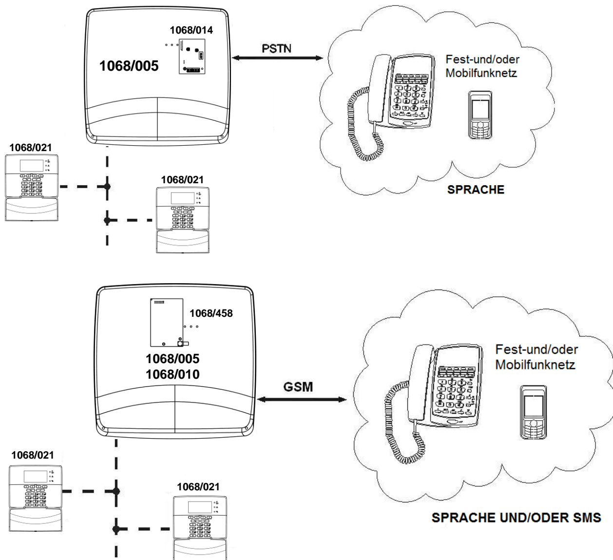
Abbildung 2 - Diagramm für die Verbindung an standortferne Benutzer
