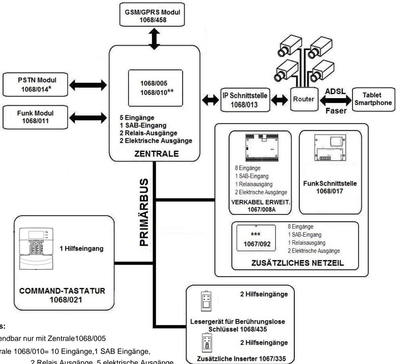
Abbildung 1 - Architektur von Systems der Serie 1068
