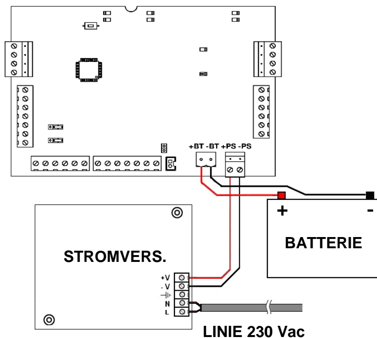
Abbildung 9 - Anschluss des Netzteils und der Batterie
