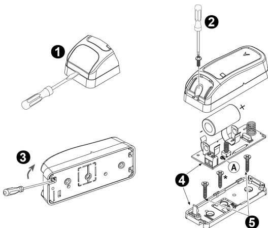
Abb. 3a. Melder montieren.
